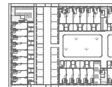
begane grond
